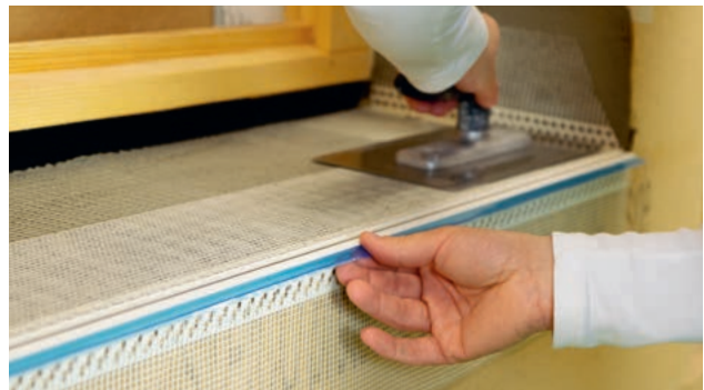
10 Einbau: Gewebeeckwinkel seitlich (optional), Gewebeeinlage flächig, STEICO secure Abschlussprofil FB an die Vorderkante
