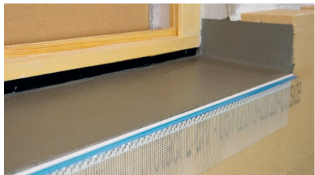
11 Das Gewebe mit STEICO secure Base Guard überziehen
